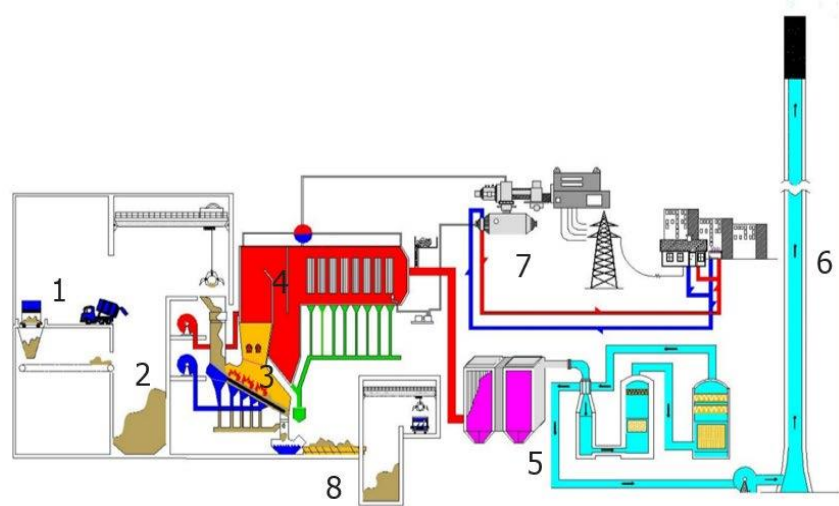
Gambar 7.7 Elemen Utama Sarana PSEL
