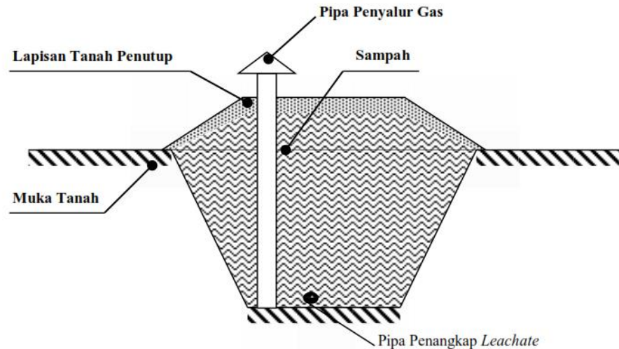
Gambar 2.9 Pengolahan Sampah Controlled Landfill di TPA
