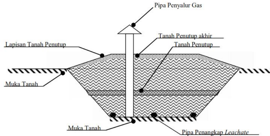
Gambar 2.10 Pengolahan Sampah Sanitary Landfill Di TPA Sumber: Damanhuri (1994)
