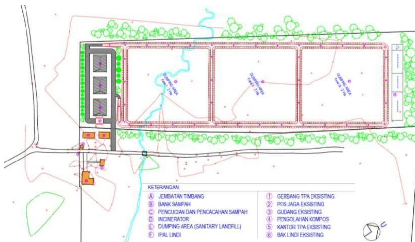
Gambar 7.6 Layout Perluasan TPA Iwaka
